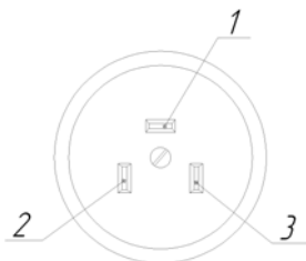
Рис. 1. Подключение розетки
