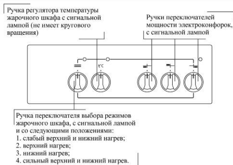
Рис. 8. Передняя панель плиты ЭП 301СТ
