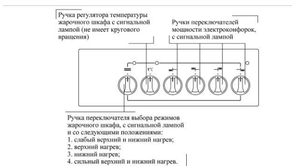
Рис. 7. Передняя панель плиты ЭП 401СТ
