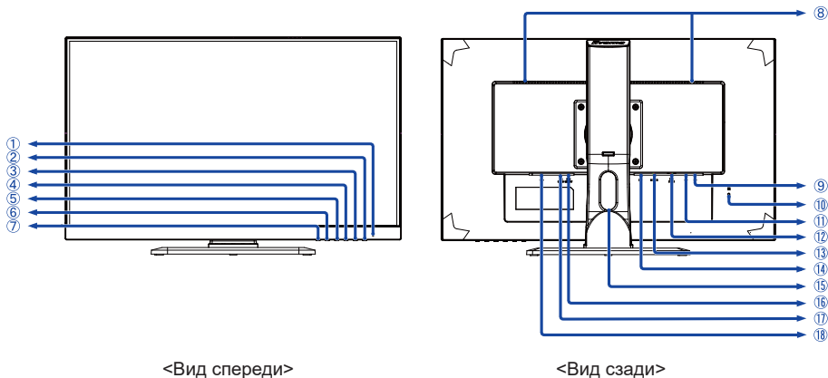
<Вид спереди>
